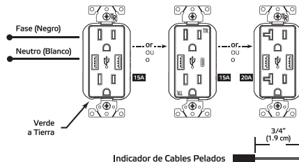
Diagrama de Alambrado
